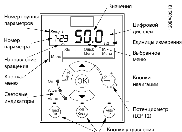
Рисунок 1.7 Описание кнопок и дисплея панели LCP
