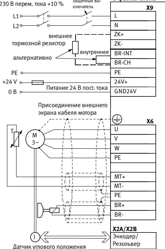
Fig. 4.2 CMMP-AS-...-3A-M3: подключение по 2-фазной схеме L1/L2 к источнику питания и мотору
