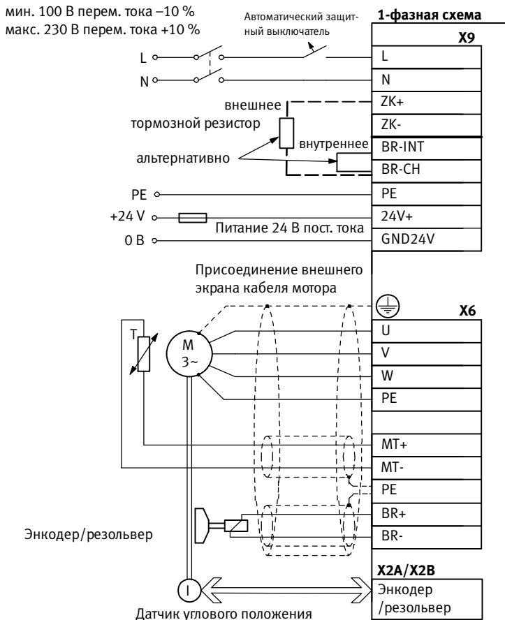
Fig. 4.1 CMMP-AS-...-3A-M3: подключение по 1-фазной схеме к источнику питания и мотору
