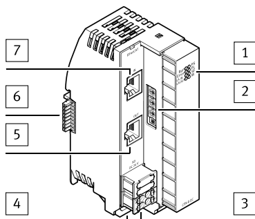
Fig. 1 Конструкция изделия
