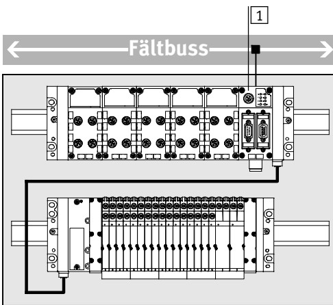
Fig. 6: Bussnodsposition höger (exempel)
