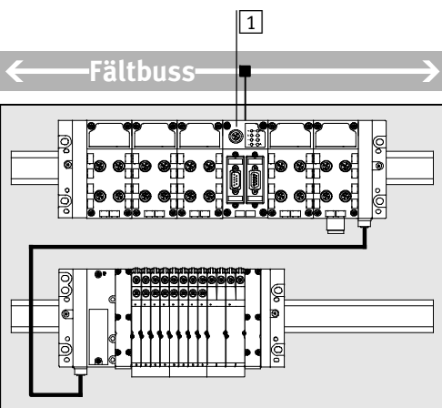
Fig. 7: Valfri bussnodsposition (exempel)
