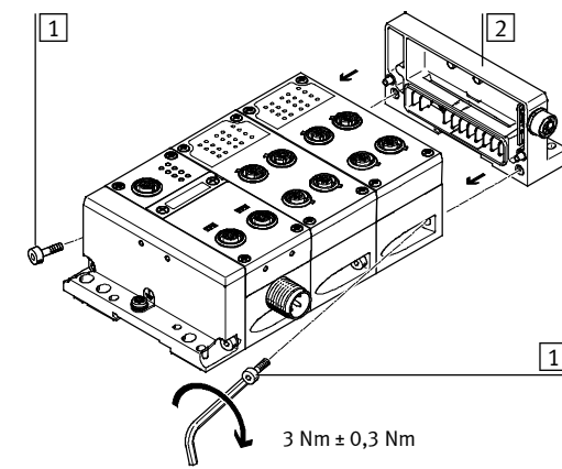
Fig. 12: Montera höger ändplatta, metallutförande
