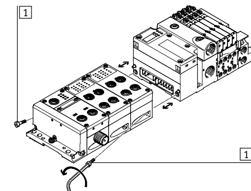
Fig. 11: Dela en CPX-terminal, metallutförande
