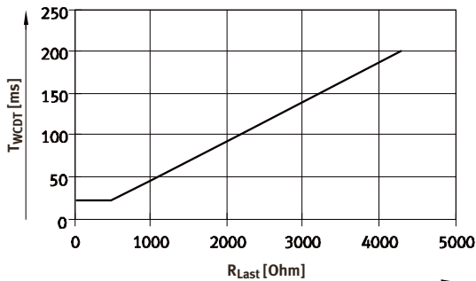
Fig. 6 Внутреннее время реакции в зависимости от значения минимальной омической нагрузки
