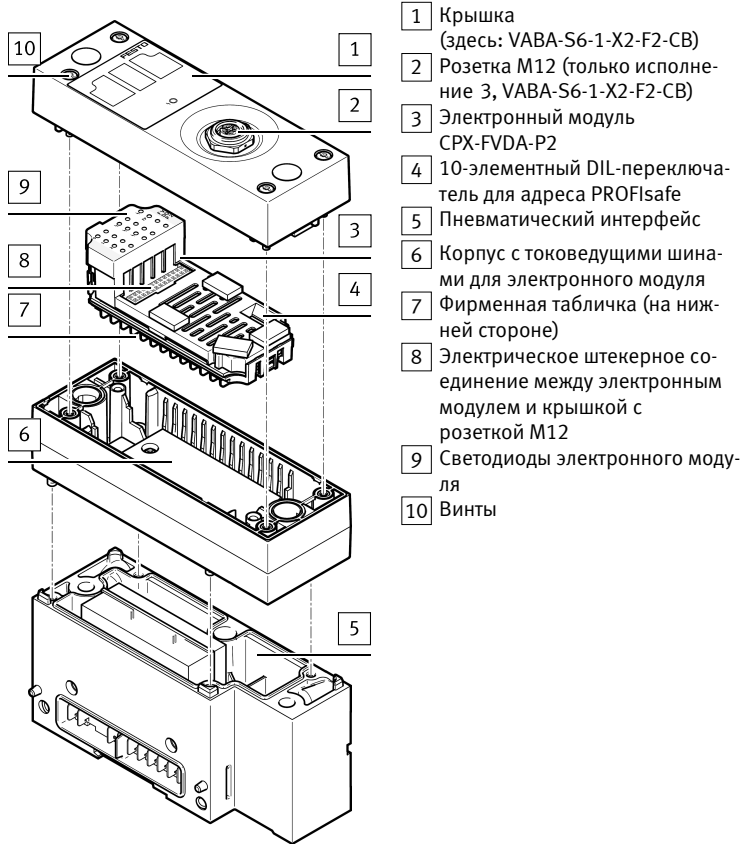
Fig. 2 Модуль выходов CPX-FVDA-P2 в пневматическом интерфейсе VABA-S6-1-X...-F1/F2-CB пневмоострова VTSA-F-CB
