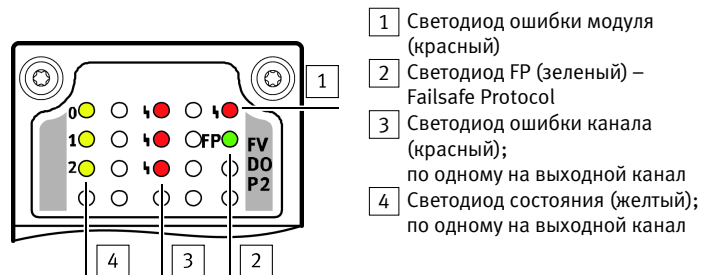
Fig. 3 Светодиодная индикация модуля выходов CPX-FVDA-P2
