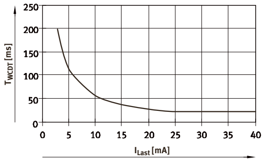
Fig. 5 Внутреннее время реакции в зависимости от значения тока минимальной нагрузки
