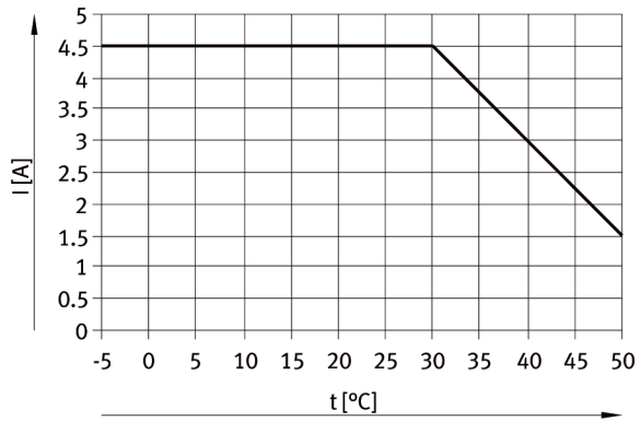
Fig. 7 Зависимость максимального выходного тока от температуры окружающей среды (во время эксплуатации) при использовании модуля выходов в пневматическом интерфейсе VABA-S6-1-X...-F1/F2-CB
