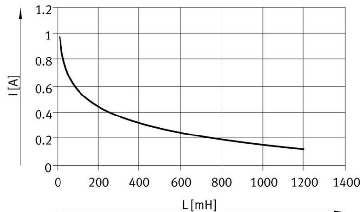
Fig. 4 Максимально допустимая индуктивность нагрузки на выходных каналах
