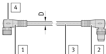
Fig. 4 NEBU-M8W3...-M8W...
