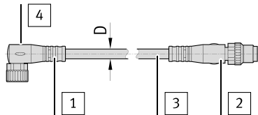
Fig. 3 NEBU-M8W3...-M8G...
