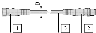
Fig. 1 NEBU-M8G3...-M8G...
