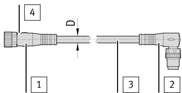
Fig. 2 NEBU-M8G4...-M8W...
