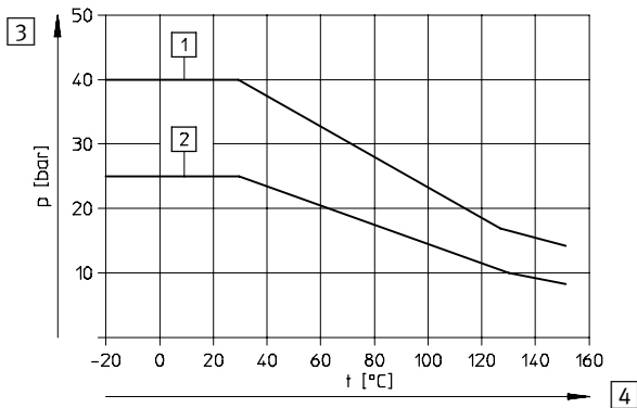
图 4: 压力温度曲线
