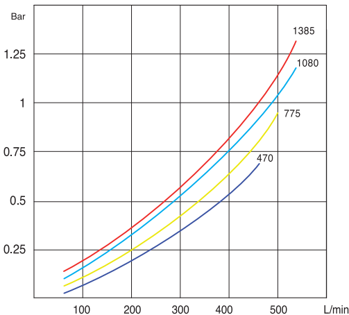
Расходно-перепадная характеристика
