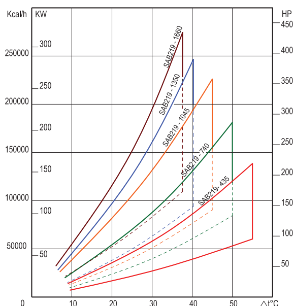
Диаграмма отводимой мощности
