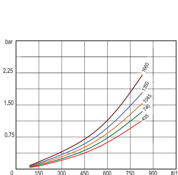
Расходно-перепадная характеристика
