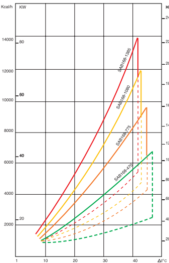
Диаграмма отводимой мощности
