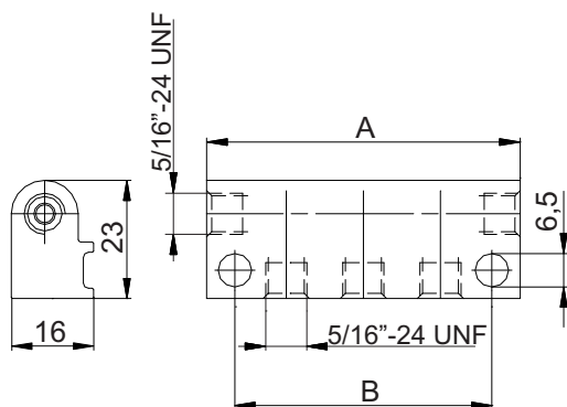
Коллекторы с выходами в одну сторону
