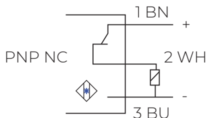
Схема подключения
