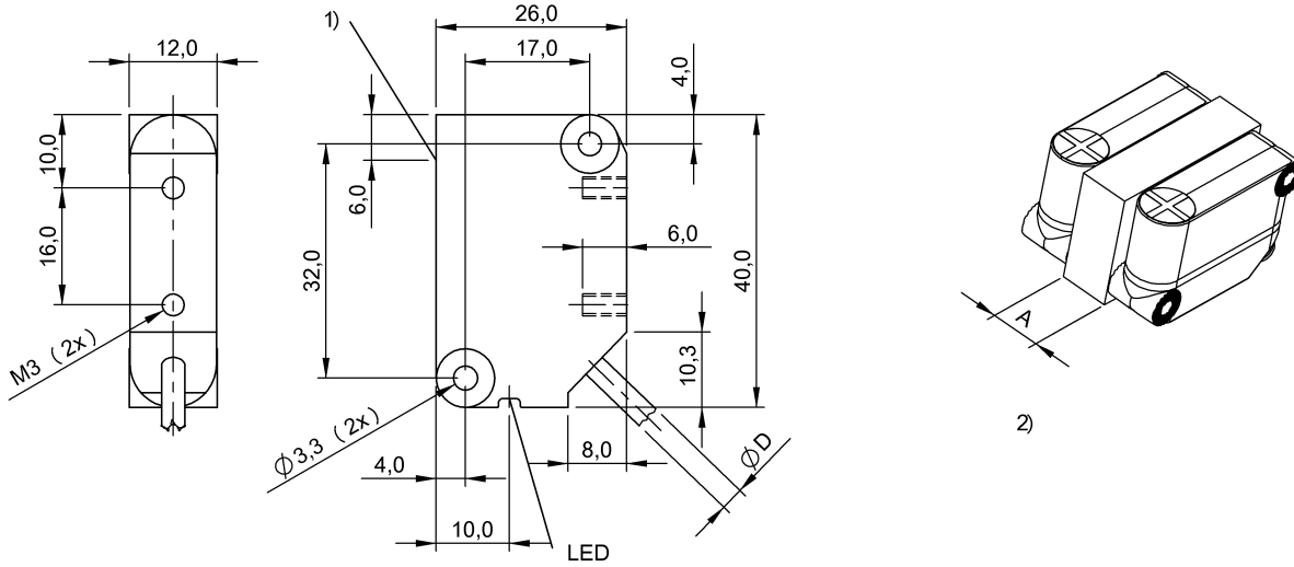
1) Активная поверхность Ø8 2) См. примечания
