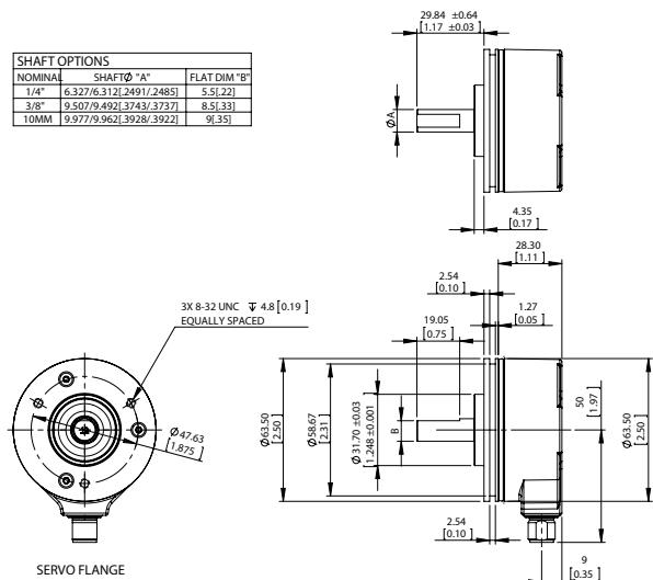
SERVO FLANGE
