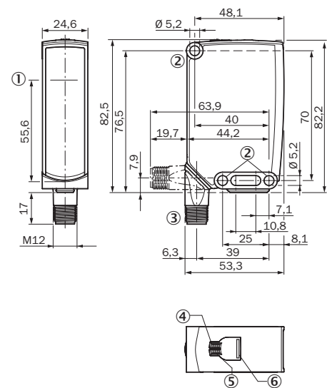
Figura 72: Dibujo acotado 2, conector macho
