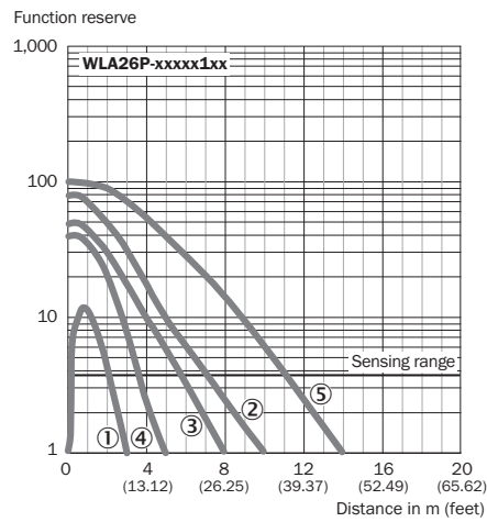
Illustration 33: Caractéristique 4 : réflecteur résistant aux produits chimiques
