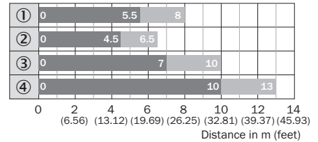
Illustration 32: Diagramme à barres 3 : réflecteurs triple fin
