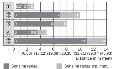
Figura 46: Diagrama de barras 4: refletor resistente a químicos
