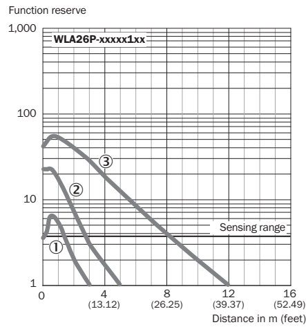
Figura 65: Curva característica 2: lámina de reflexión
