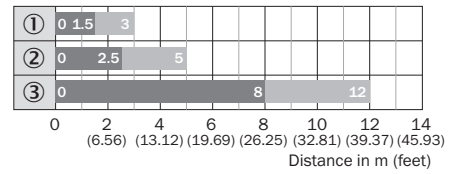
Illustration 30: Diagramme à barres 2 : bande réflecteur
