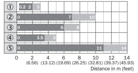
插图 82: 条形图 4: 耐化学性反射器
