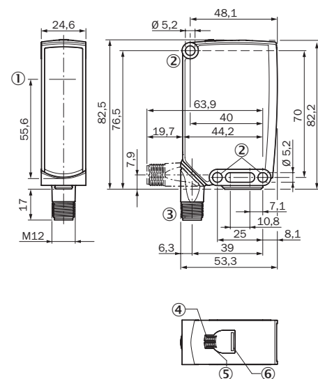
Figura 60: Disegno quotato 2, connettore maschio
