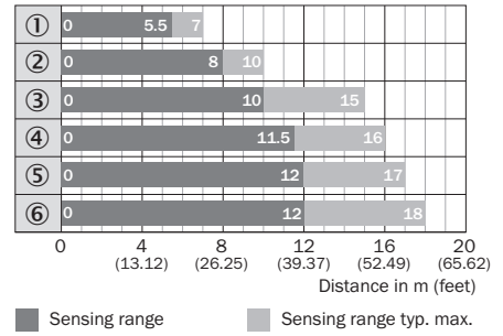
Figura 64: Gráfico de barras 1: reflector estándar
