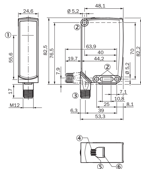
Abbildung 24: Maßzeichnung 2, Stecker
