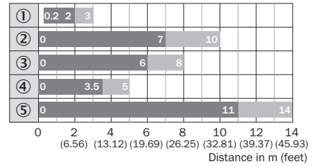
Figura 58: Diagramma a barre 4: riflettore resistente alle sostanze chimiche
