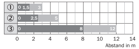
Abbildung 18: Balkendiagramm 2: Reflexionsfolie
