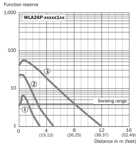
Figura 53: Linea caratteristica 2: riflettore adesivo
