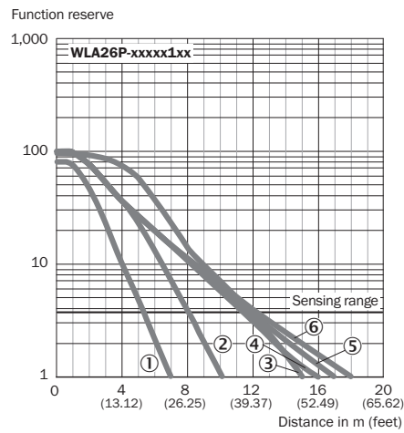
Figura 39: Curva característica 1: refletor padrão
