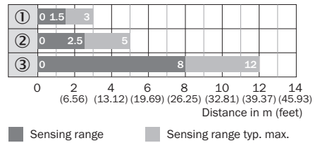
Figura 42: Diagrama de barras 2: fita refletiva
