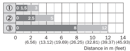
図 90: 棒グラフ 2: 反射テープ
