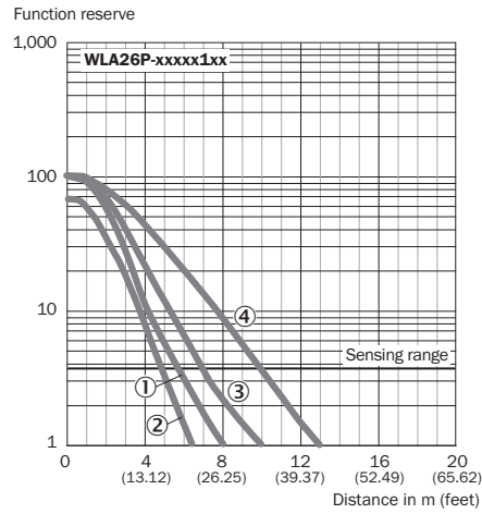
Рисунок 103: Характеристика 3: высококачественные тройные отражатели
