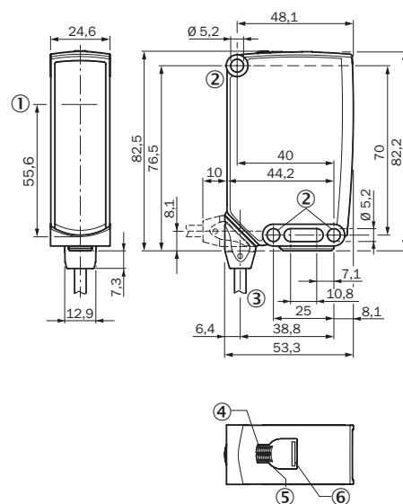
Figura 59: Disegno quotato 1, cavo
