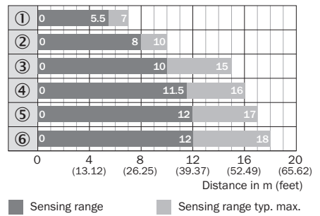
Figura 40: Diagrama de barras 1: refletor padrão
