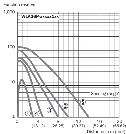
Figura 45: Curva característica 4: refletor resistente a químicos
