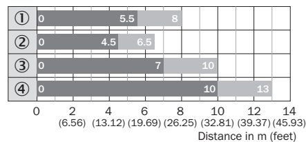
図 92: 棒グラフ 3: 高精度トリプルリフレクタ
