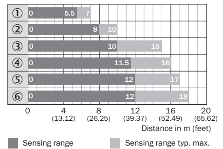
Figura 52: Diagramma a barre 1: riflettore standard
