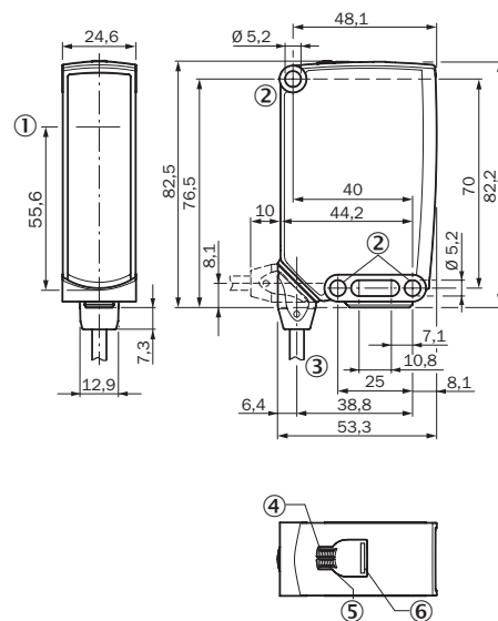
Рисунок 107: Масштабный чертёж 1, кабель
