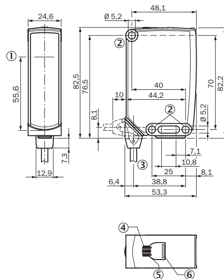
插图 83: 尺寸图 1, 电缆
