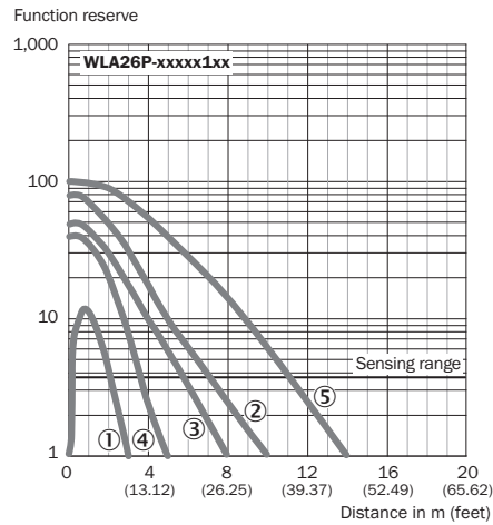
Рисунок 105: Характеристика 4: химически стойкий отражатель
