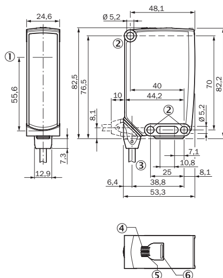
図 95: 寸法図 1、ケーブル
