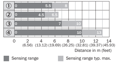
Рисунок 104: Столбиковая диаграмма 3: высококачественные тройные отражатели
