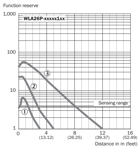
図 89: 特性曲線 2: 反射テープ
