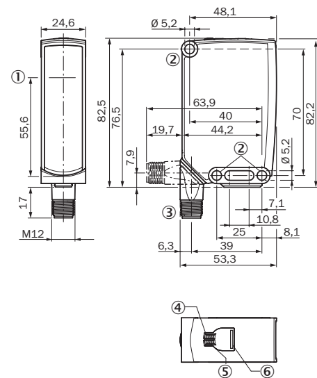
插图 84: 尺寸图 2, 插头
