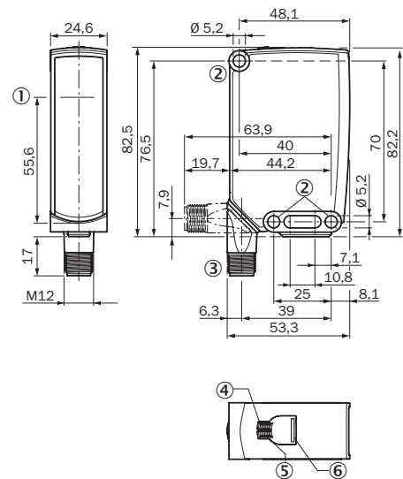
Figura 48: Desenho dimensional 2, conector macho
