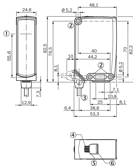
Figura 71: Dibujo acotado 1, cable
