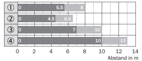
Abbildung 20: Balkendiagramm 3: Feintripple Reflektoren
