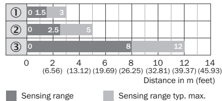
插图 78: 条形图 2: 反光膜
