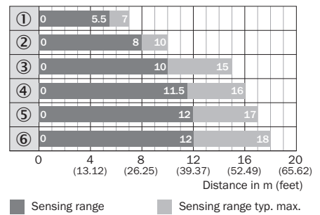
Illustration 28: Diagramme à barres 1 : réflecteur standard
