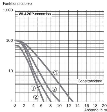
Abbildung 19: Kennlinie 3: Feintripple Reflektoren
