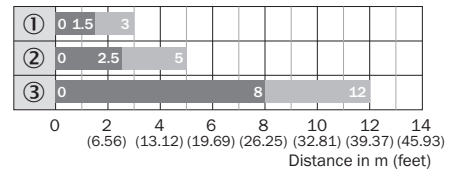
Рисунок 102: Столбиковая диаграмма 2: отражающая плёнка
