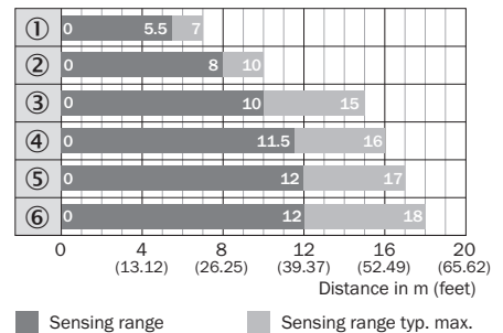
插图 76: 条形图 1: 标准反射器
