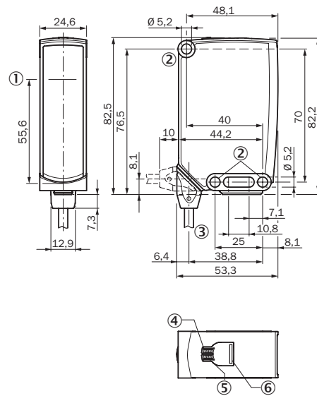
Figura 47: Desenho dimensional 1, cabo
