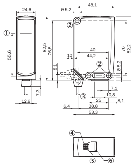
Illustration 35: Plan coté 1, câble
