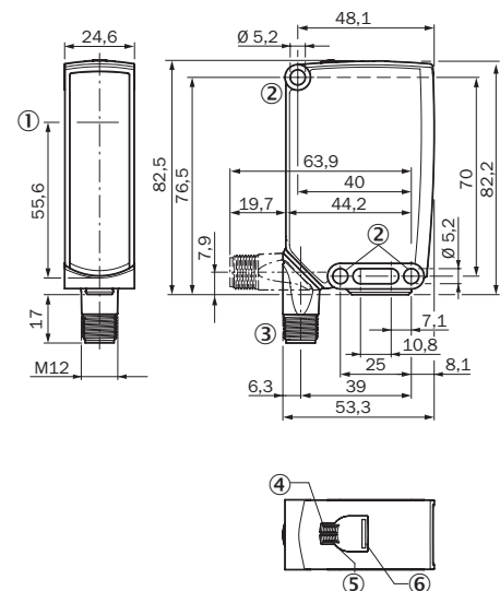
Рисунок 108: Масштабный чертёж 2, штекер
