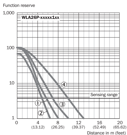
插图 79: 特征曲线 3: 高精三重反光镜
