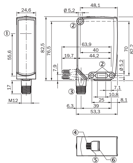
図 96: 寸法図 2、オスコネクタ
