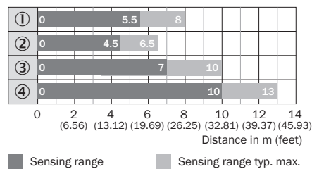
插图 80: 条形图 3: 高精三重反光镜
