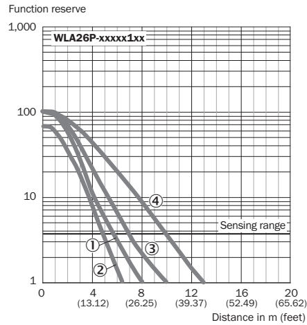
Figura 55: Linea caratteristica 3: riflettori a microprismi
