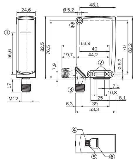
Illustration 36: Plan coté 2, connecteur mâle
