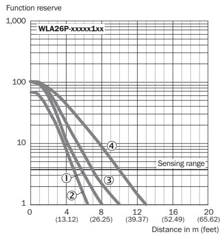
Figura 43: Curva característica 3: refletores com espelhos prismáticos finos
