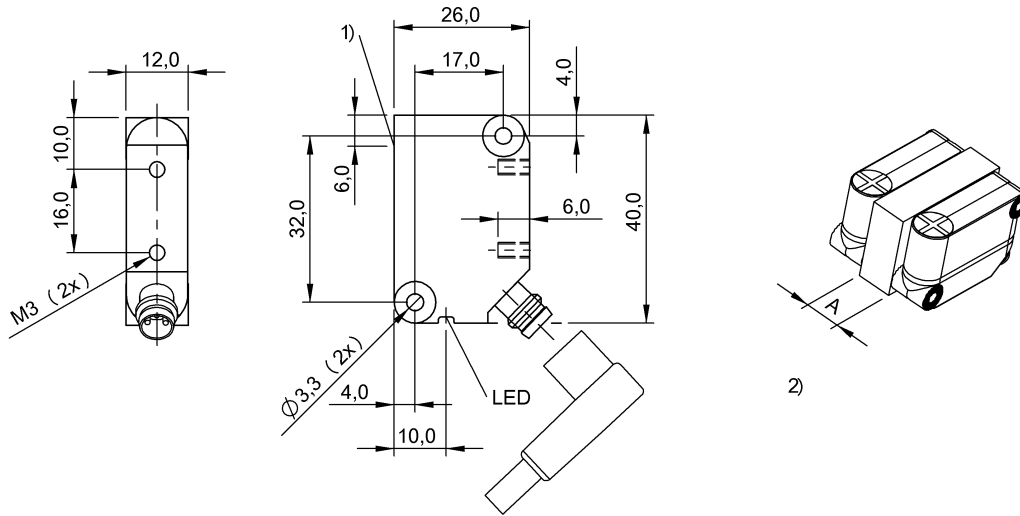
1) Активная поверхность Ø8 2) См. примечания
