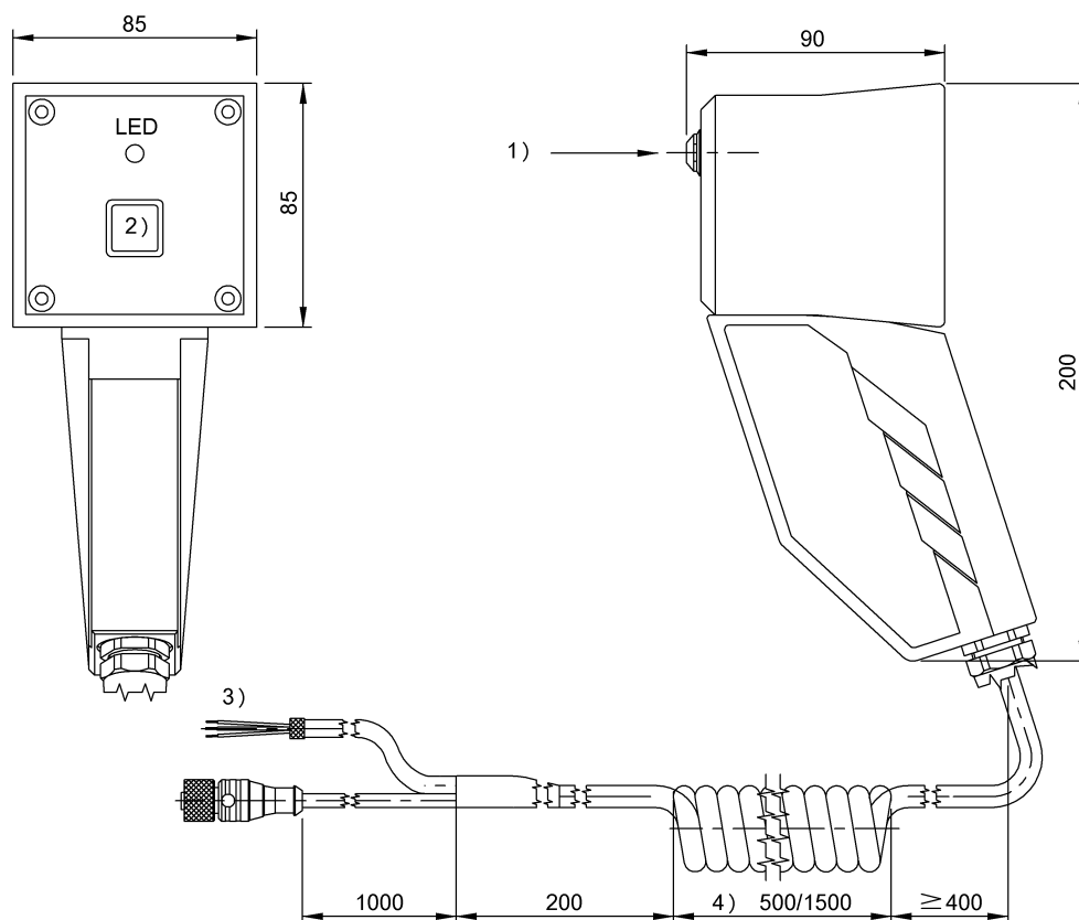
1) см. примечания, 2) Кнопка, 3) см. схему подключения, 4) Длина сжатой / разжатой спирали
