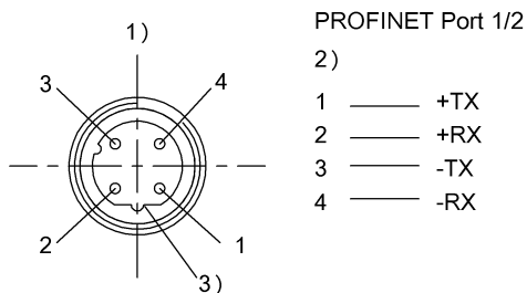
1) Вид в направлении вставки 2) Гнездо 4-конт./ функция 3) Кодировка D
