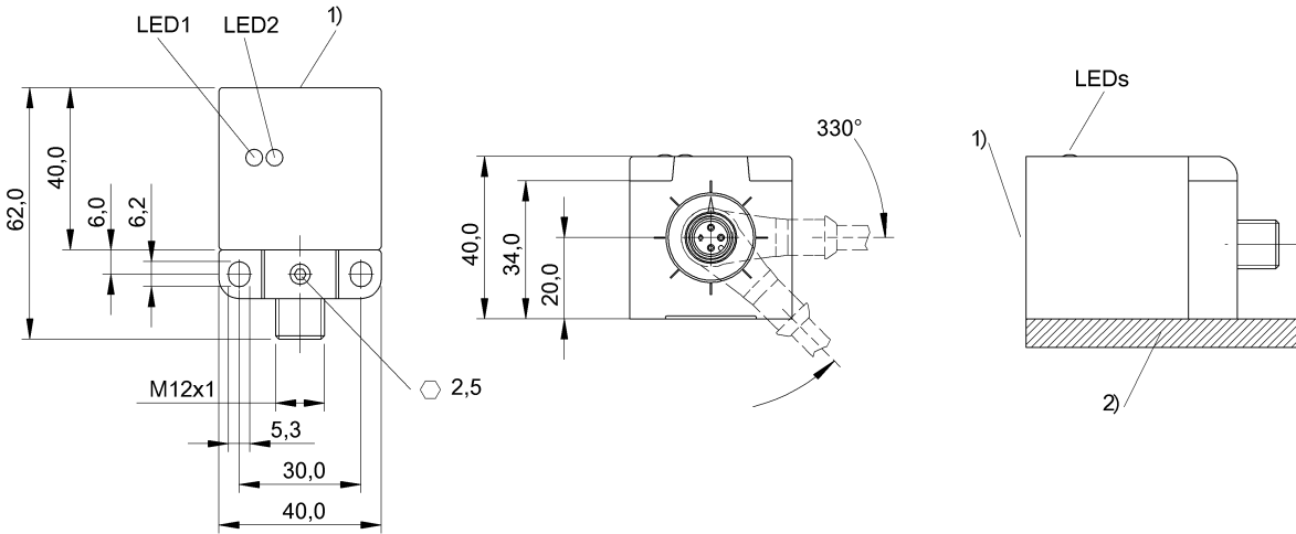
1) Активная поверхность 2) Металлическая пластина
