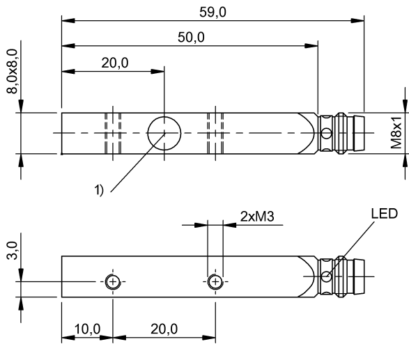
1) Активная поверхность
