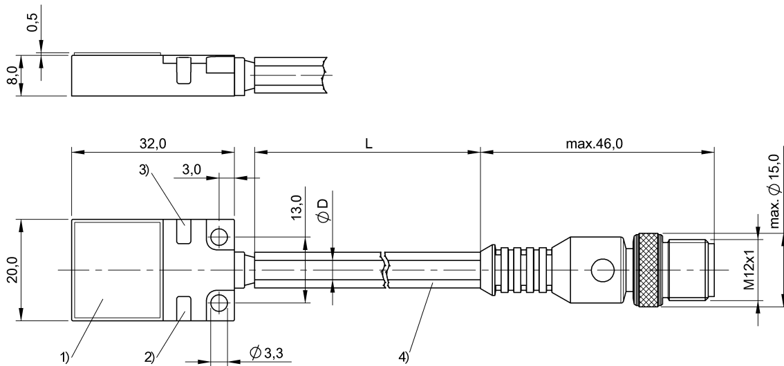
1) Активная поверхность 2) СД зеленый 3) СД желтый 4) Силиконовый шланг D = 7 мм
