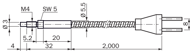
Габаритный чертёж (Размеры, мм)
