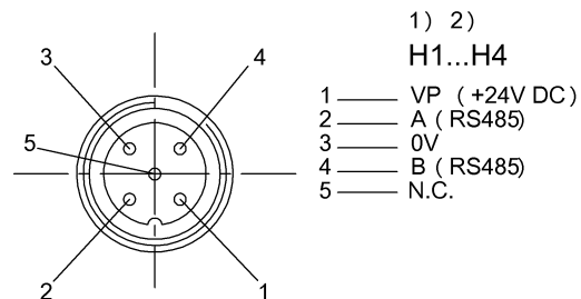
1) Вид в направлении вставки 2) Гнездо 5-конт./ функция
