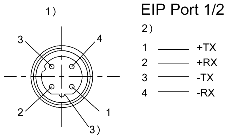
1) Вид в направлении вставки 2) Гнездо 3) Кодировка D
